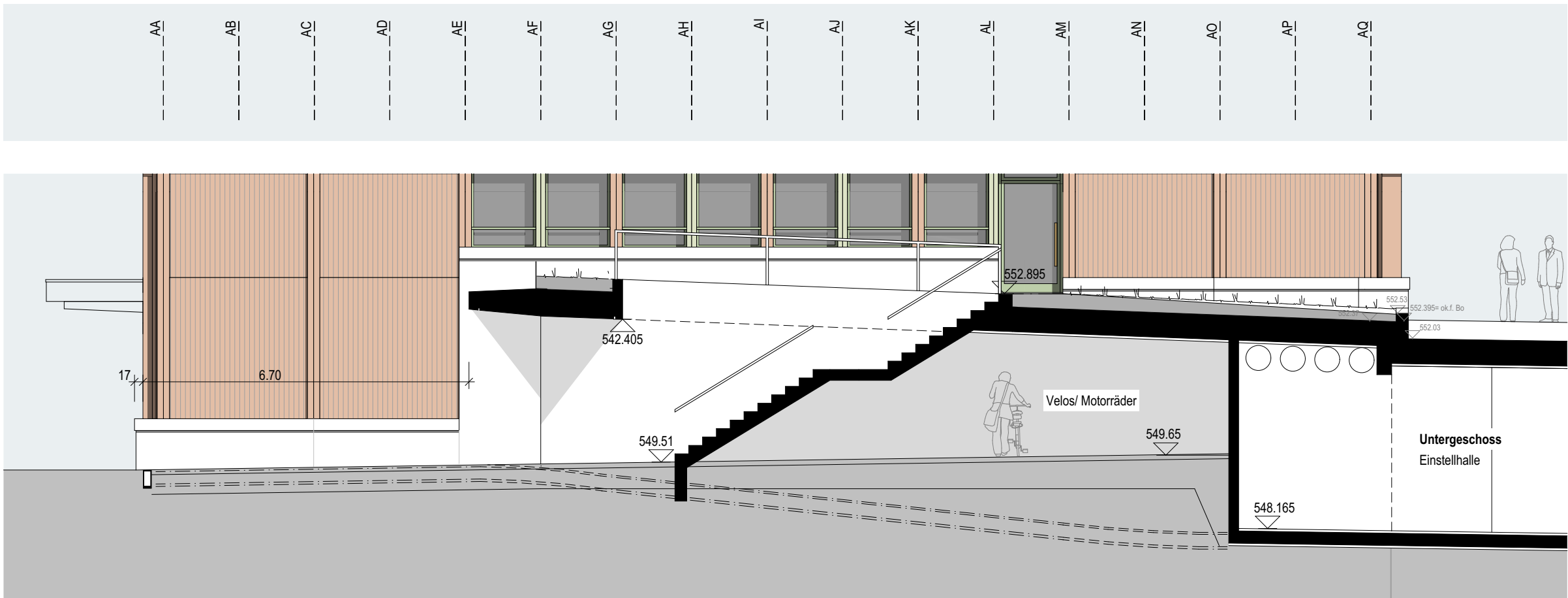
Ansicht Nord, Neubau Schnitt FF
