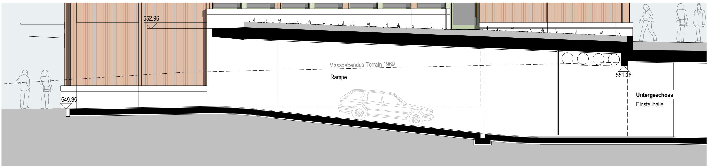
Ansicht Nord, Neubau Schnitt EE
