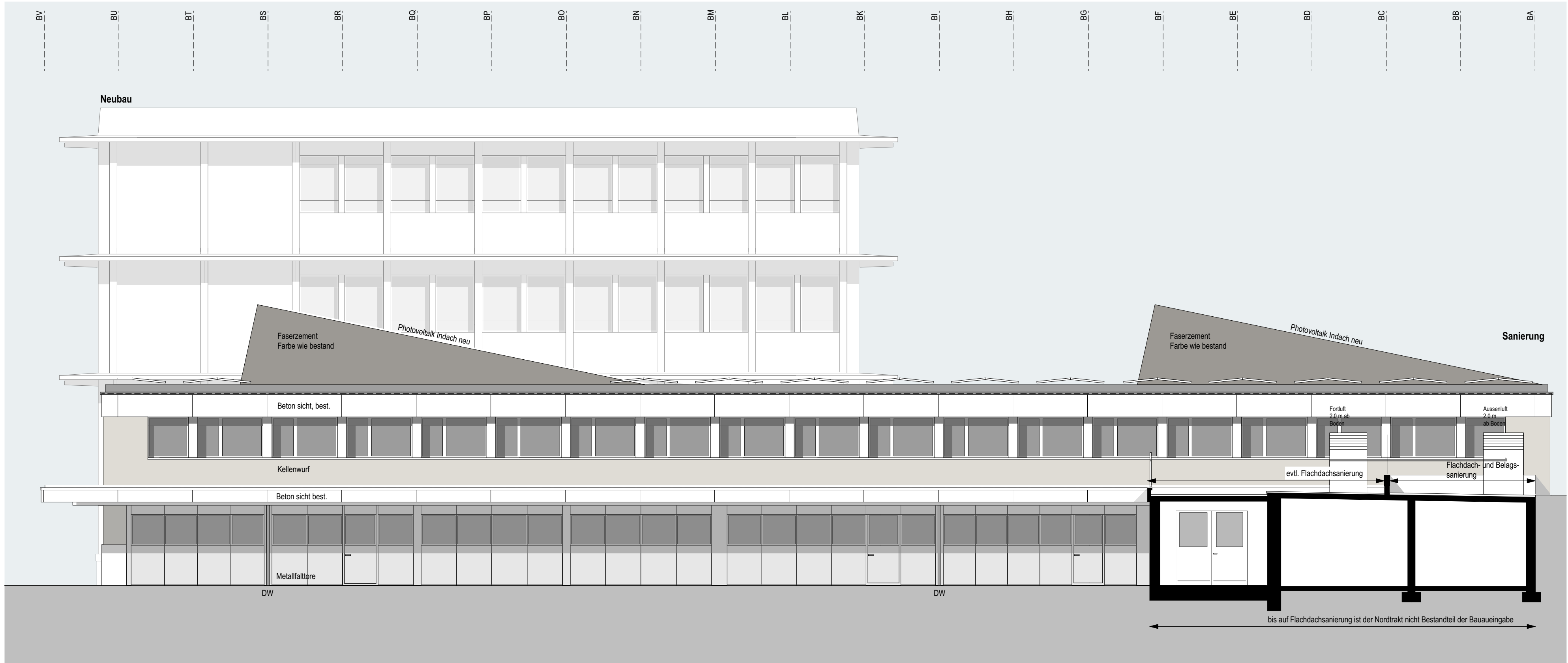
Ansicht Nord, Sanierung
